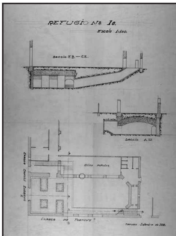
Planta i seccions del projecte del refugi núm.10 (setembre 1938)
