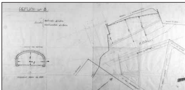
Planta i secció del projecte del refugi núm. 3 (abril 1937)
